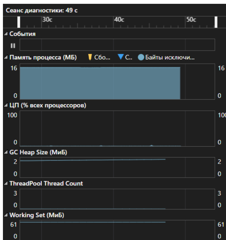
Рисунок 3.47. Производительность программы, используемые ресурсы
